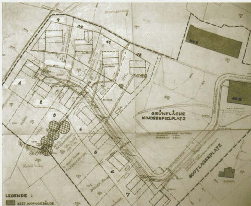
Abb. 5: Lageplan Clubsiedlung 1974
